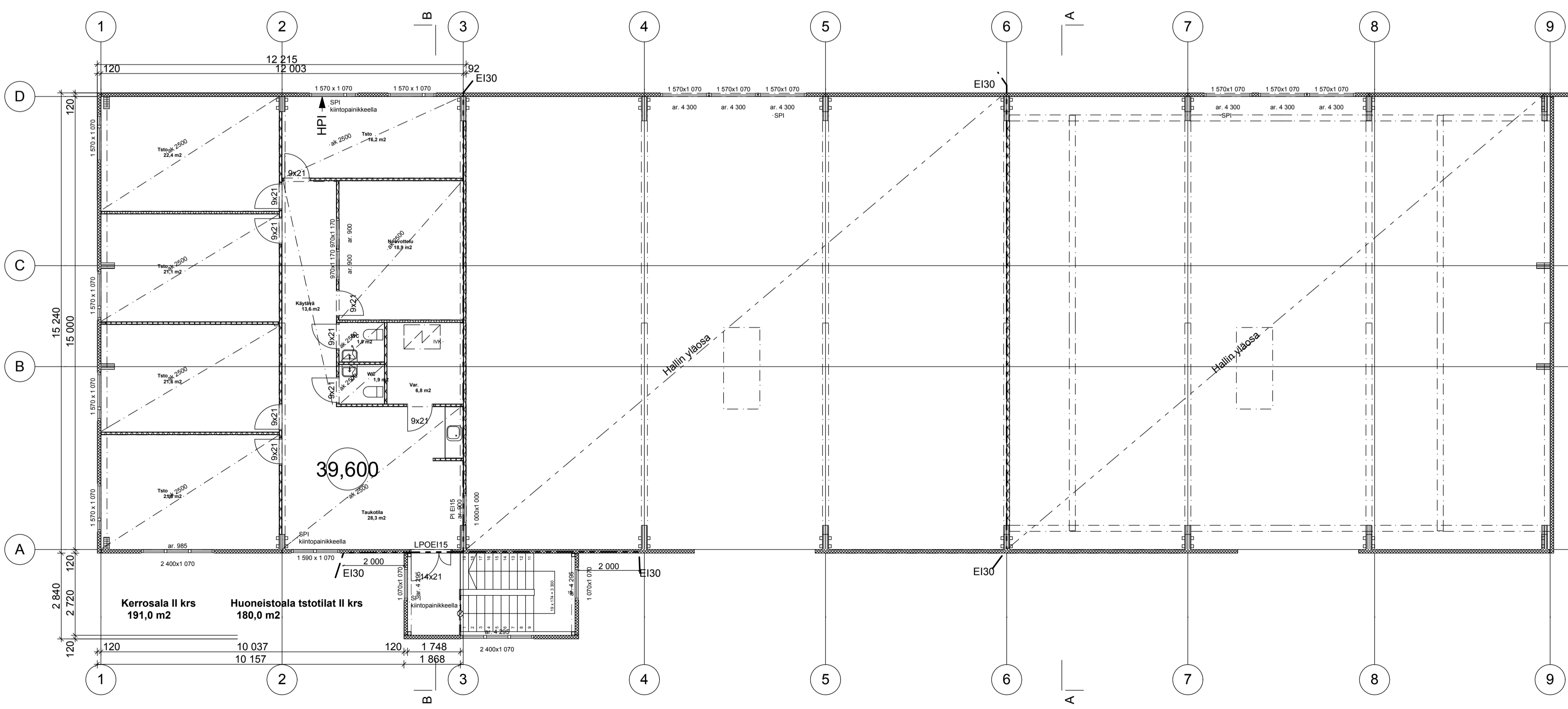
Pohjapiirustus II
