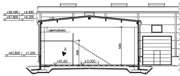
LEIKKAUS B - B 1:100
