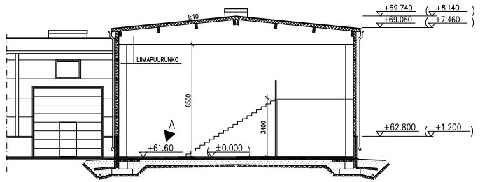
LEIKKAUS A - A 1:100
