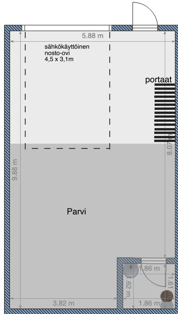
suuntaa-antava pohjakuva
